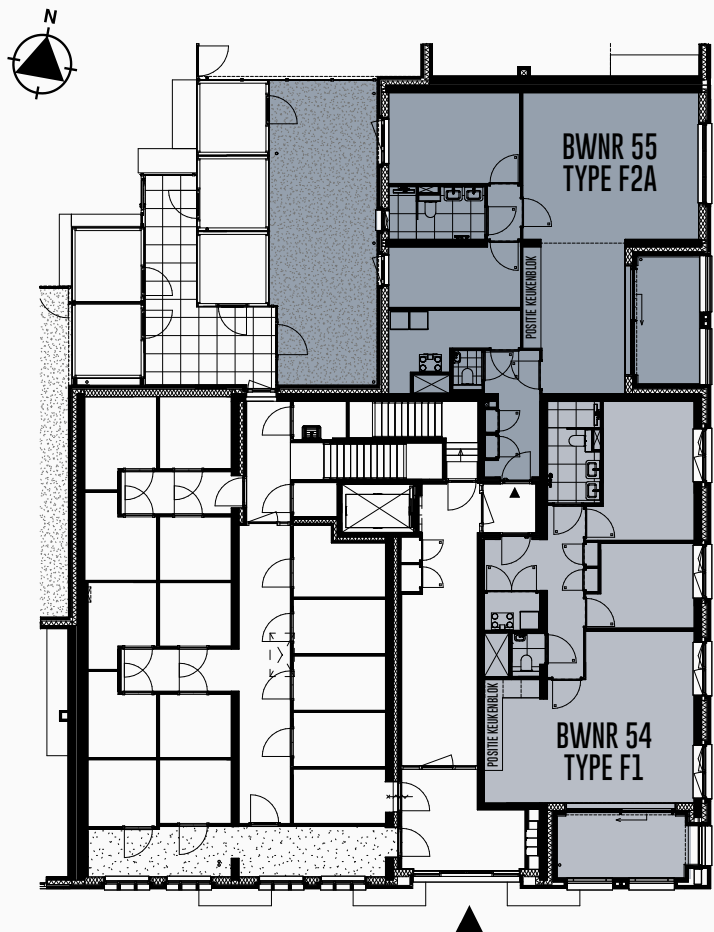
BEGANE GROND
