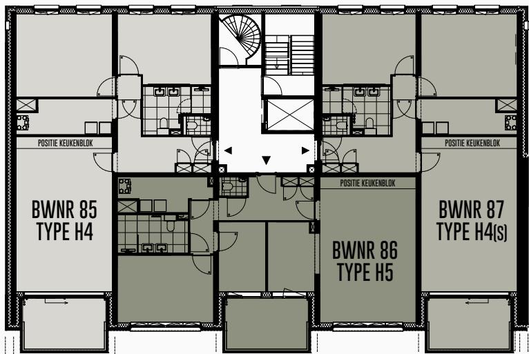
TWEDE VERDIEPING
