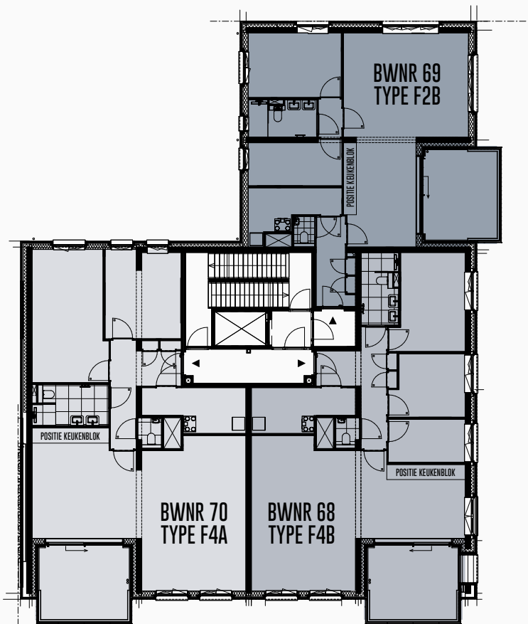
VIJFDE VERDIEPING
