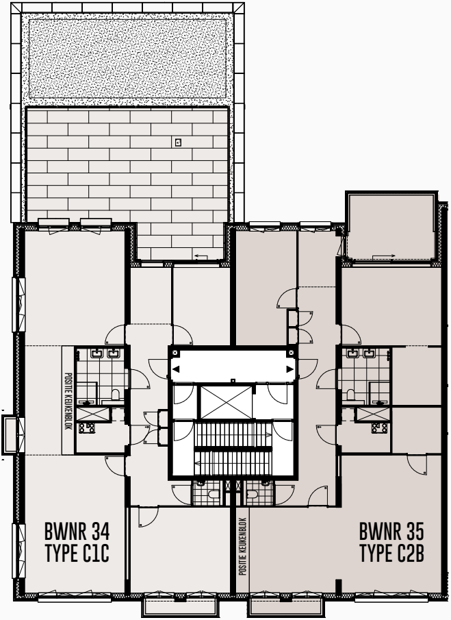
DERDE VERDIEPING
