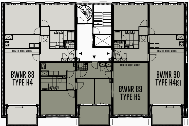
DERDE VERDIEPING
